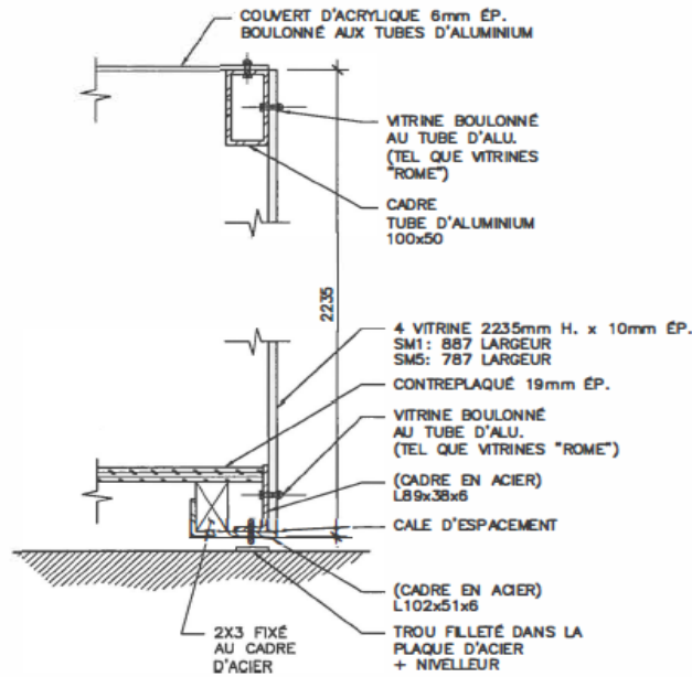
COUPE TYPIQUE ÉCHELLE: 1=5
