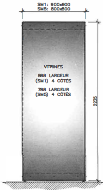
ÉLÉVATION TYPIQUE VITRINE SM1 & SM5 ÉCHELLE: 1=15
